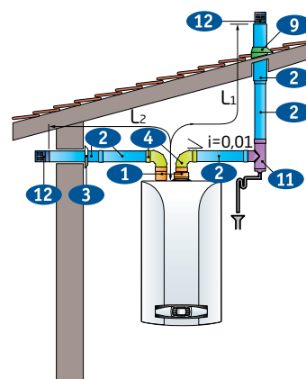
С забором воздуха через стену
