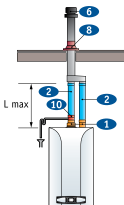
На плоскую крышу
