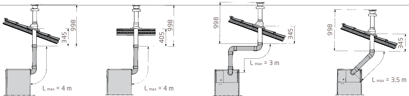
Коаксиальная труба с вертикальным выходом
