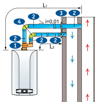
С коллективным забором воздуха
