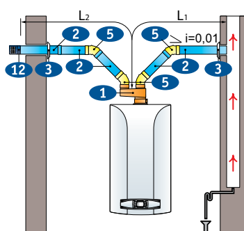
С забором воздуха с улицы
