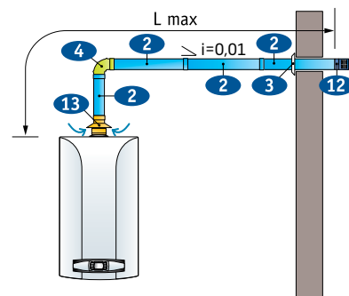
С забором воздуха из помещения
