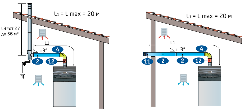
Вывод дымовой трубы в дымоход
